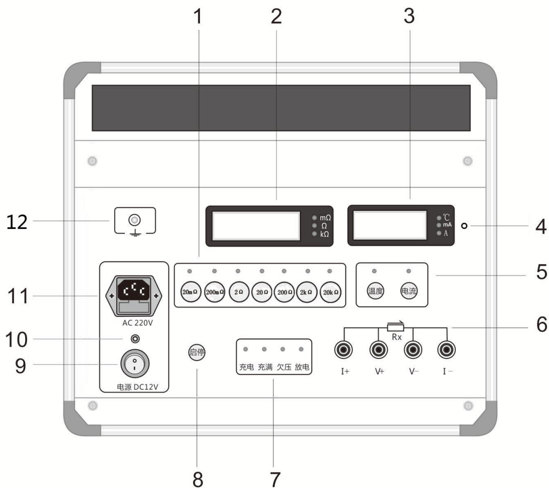
图一 面板布局图
